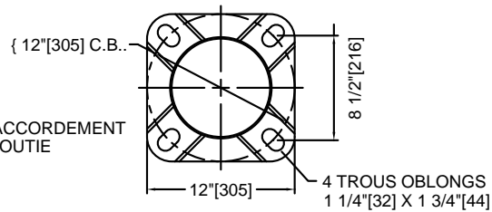
BASE D'ANCRAGE
