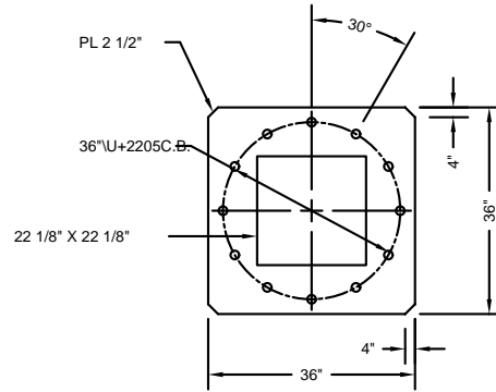
PLAQUE DE BASE (POUR B.A. 1 1/2"Ø X 81"LG)
